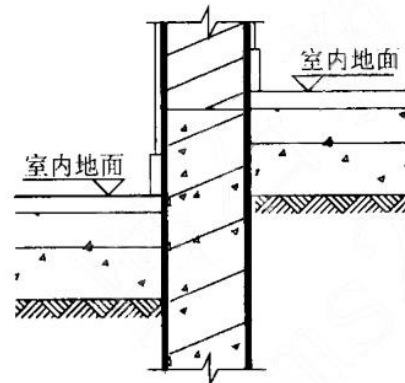
图4.2.8-4 混凝土墙基二
