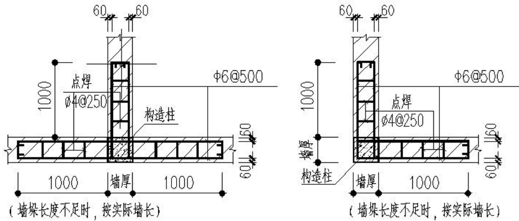
图 5.5.9 构造柱与墙拉结示意
