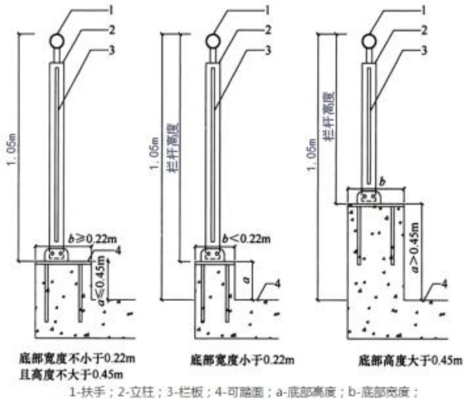
图 4.2.11-1 栏杆高度示意
