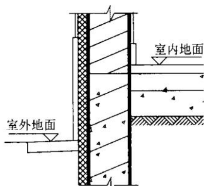
图4.2.8-3 混凝土墙基一
